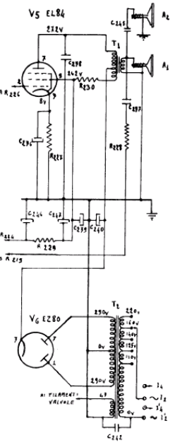
VARIANTE SU CIRCUITO DI ALIMENTAZIONE PER APPARECCHIO MODELLO 704 FC
